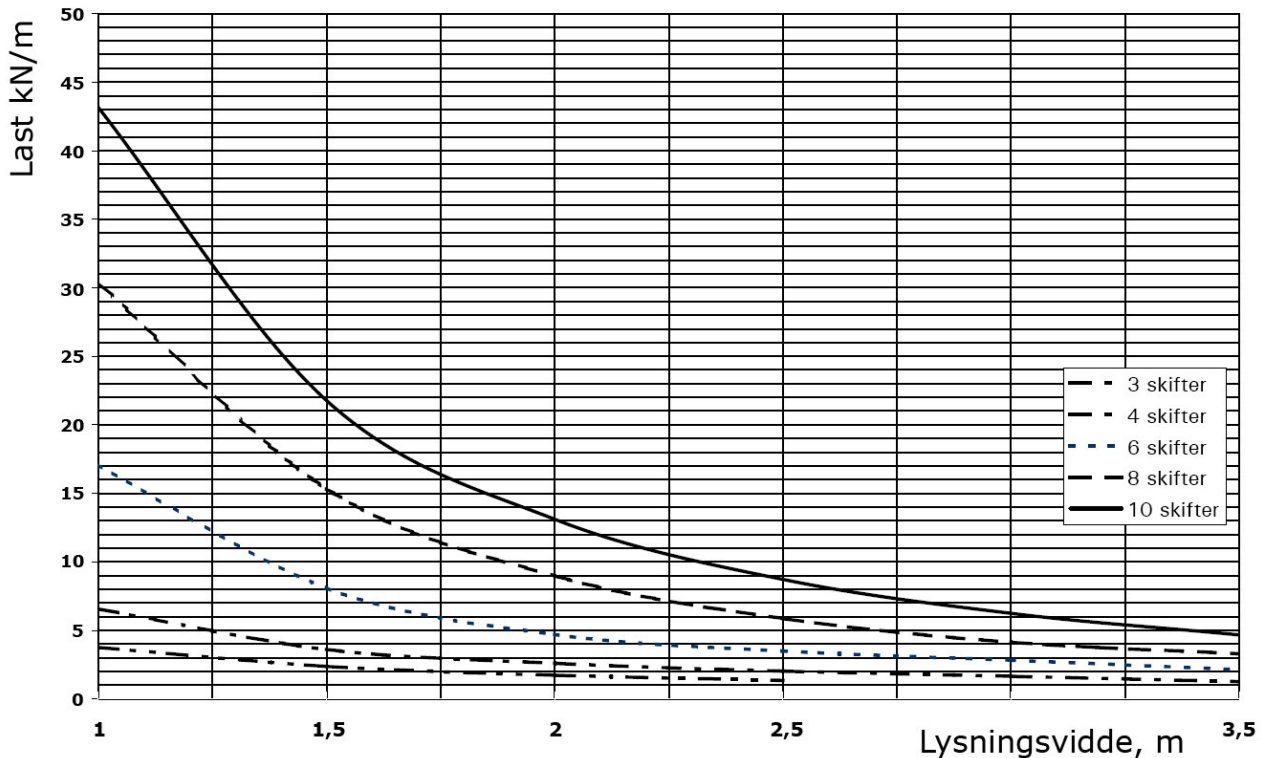
Diagram over teglbjælkens bæreevne
